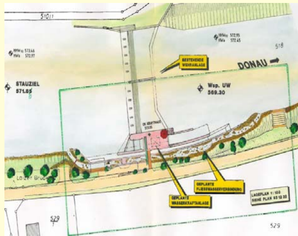
Wasserkraftwerk Laiz
