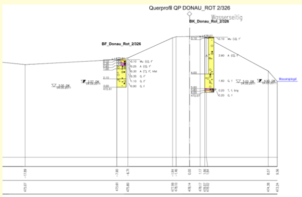
Querschnitt Damm
