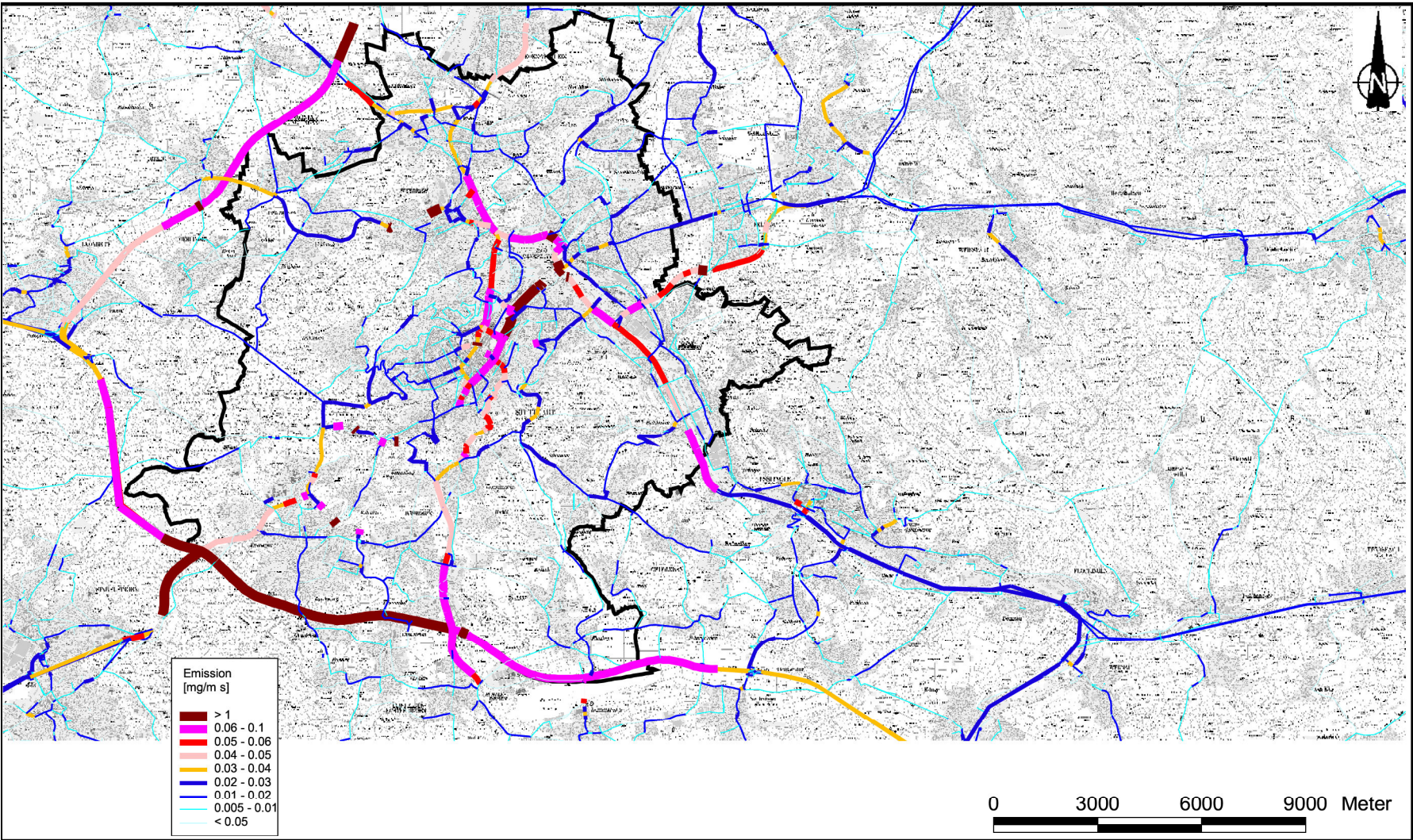
Abb. A3.3: Mittlere PM10-Emissionsdichte auf dem weitreichenden Straßennetz bei Stuttgart für den Istzustand 2010
