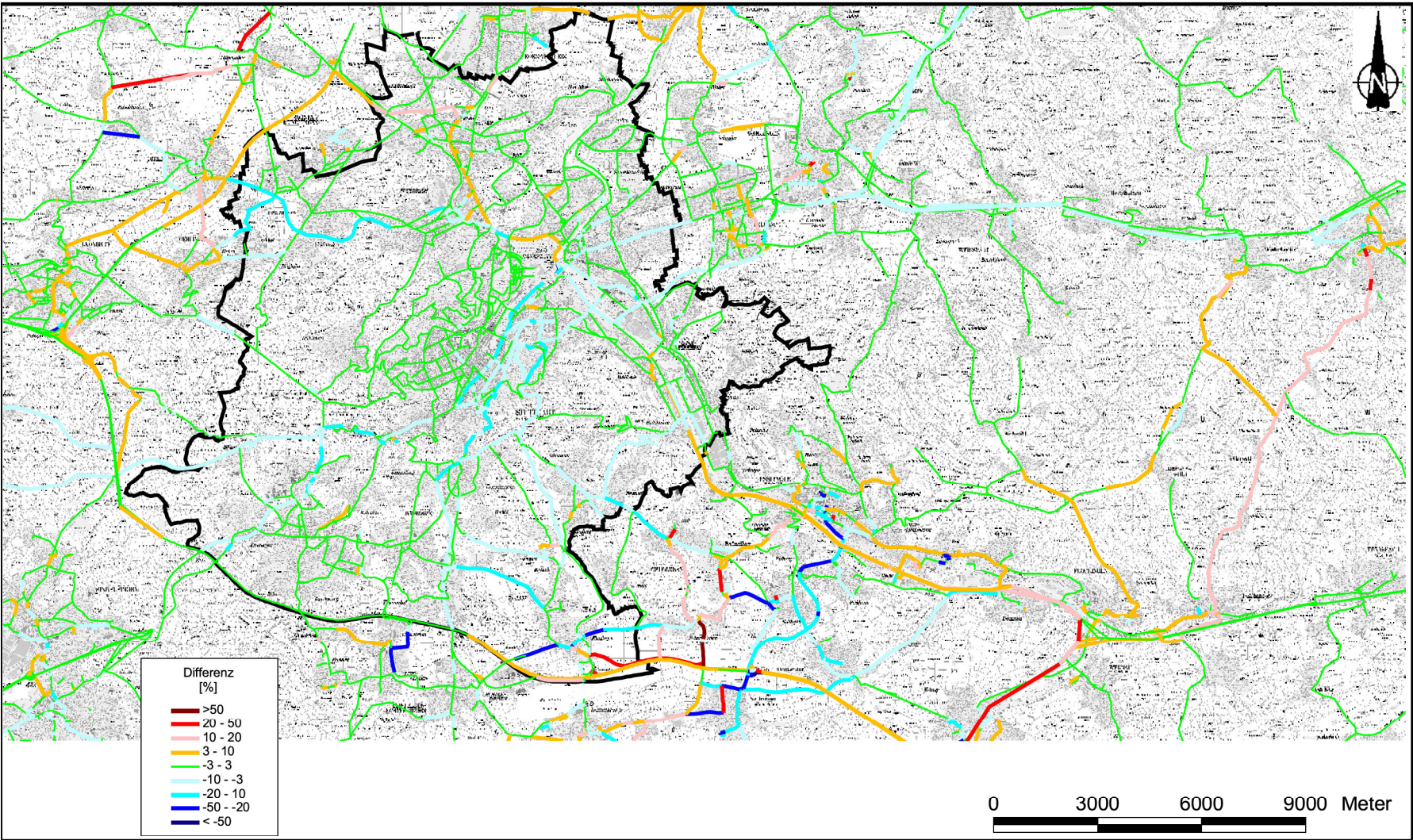
Abb. A3.2: Relative Änderung der NOx-Emissionsdichte zum Istzustand 2010 für die Maßnahme M1 im Jahr 2010 auf dem weitreichenden Straßennetz bei Stuttgart
