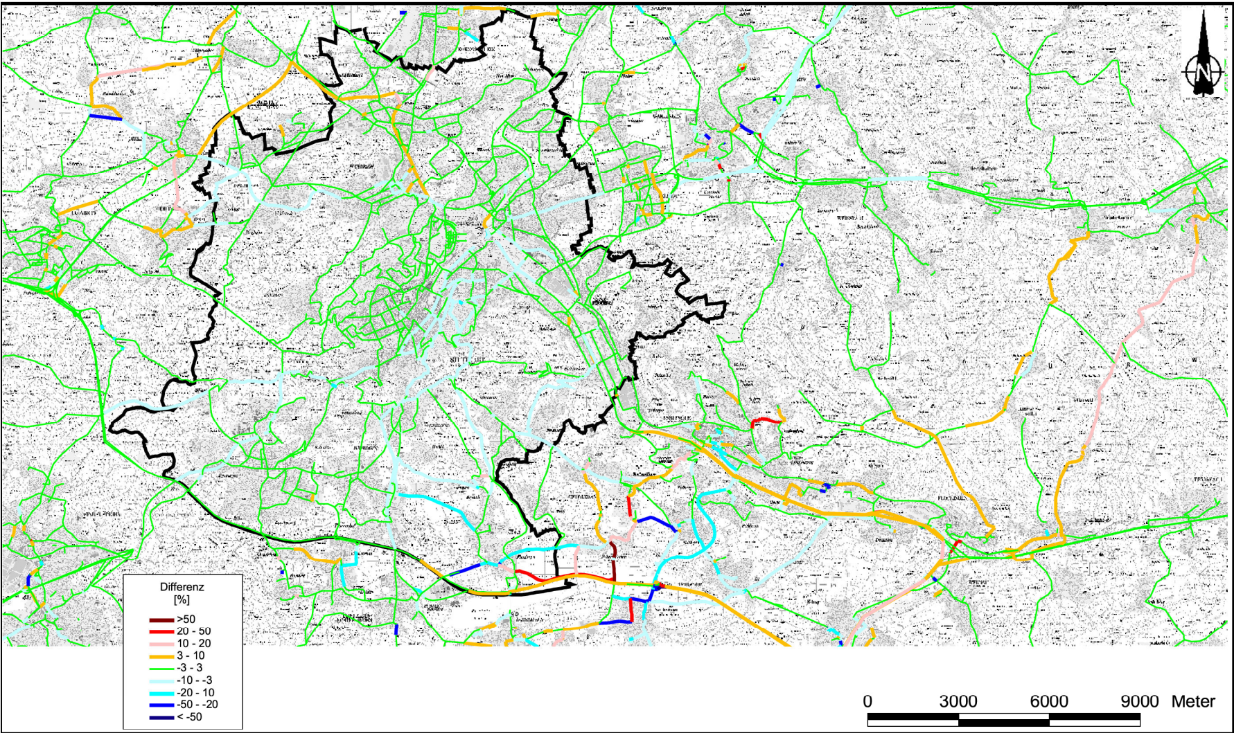
Abb. A3.4: Relative Änderung der PM10-Emissionsdichte zum Istzustand 2010 für die Maßnahme M1 im Jahr 2010 auf dem weitreichenden Straßennetz bei Stuttgart
