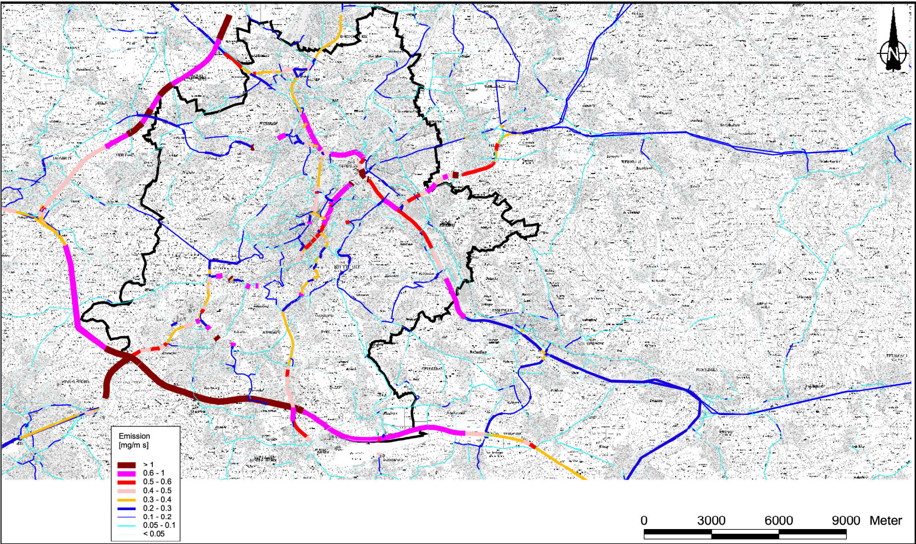
Abb. A3.1: Mittlere NOx-Emissionsdichte auf dem weitreichenden Straßennetz bei Stuttgart für den Istzustand 2010
